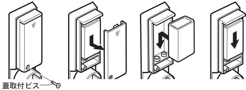
蓋取付ビス
