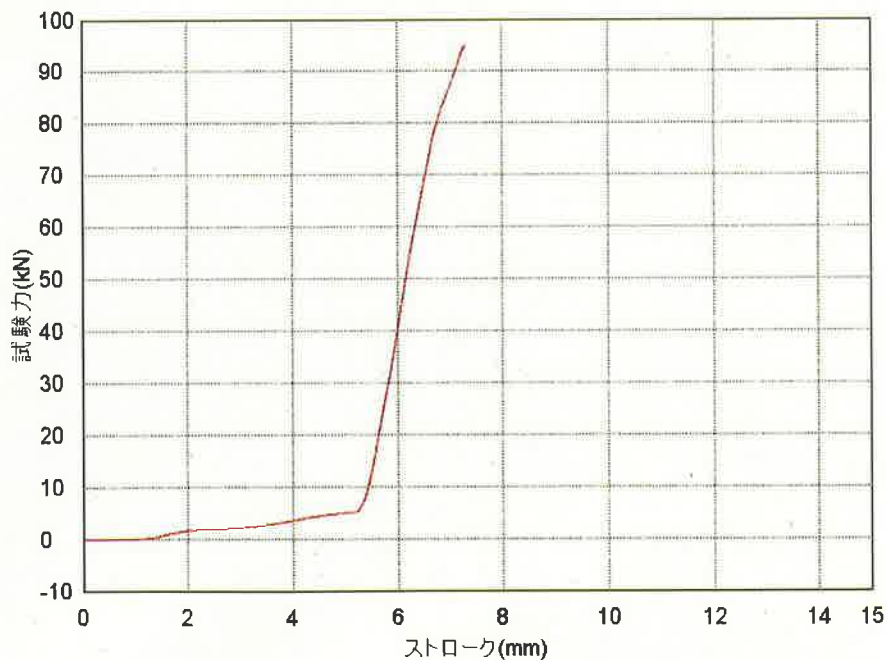
図 2 荷重-ストローク線図
